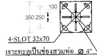
BASE PLATE ฐานเสา
